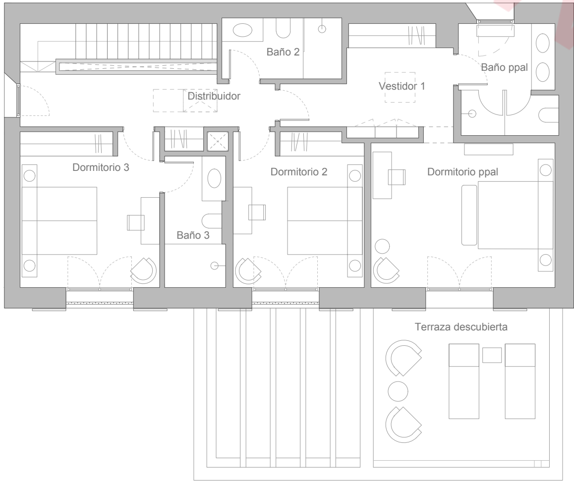
Planta Primera
