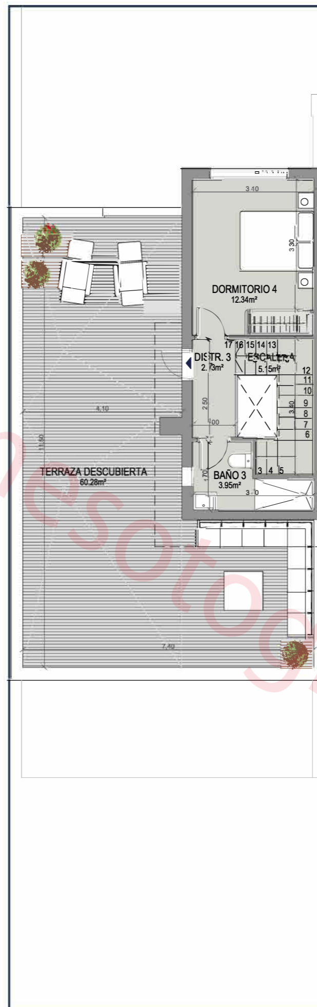
PLANTA ÁTICO
