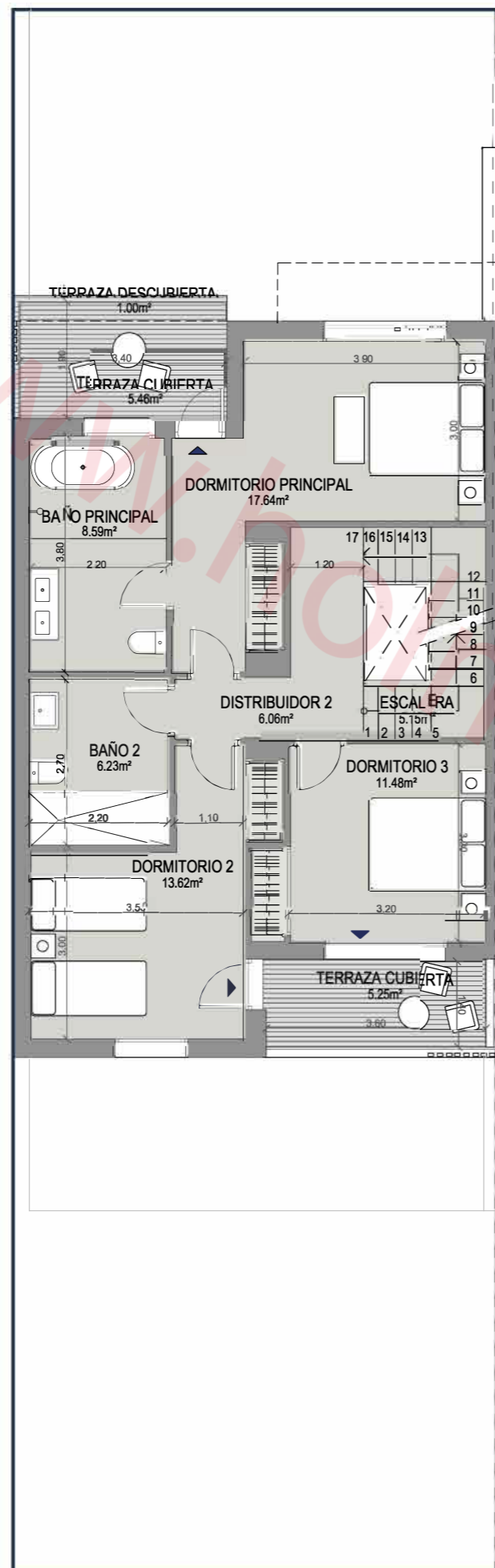
PLANTA PRIMERA
