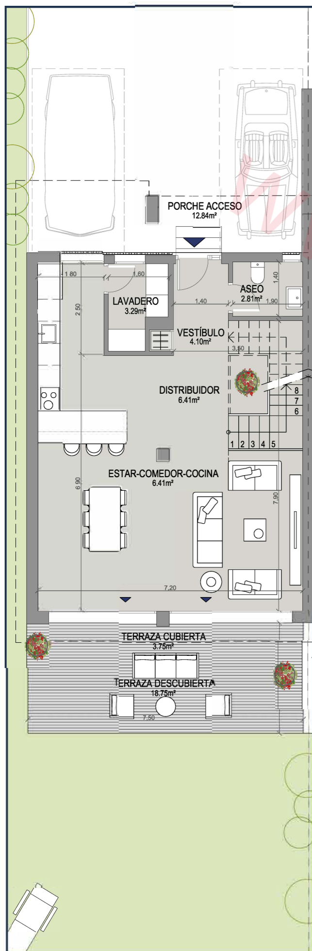
PLANTA BAJA
