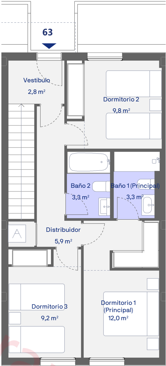
Planta primera
